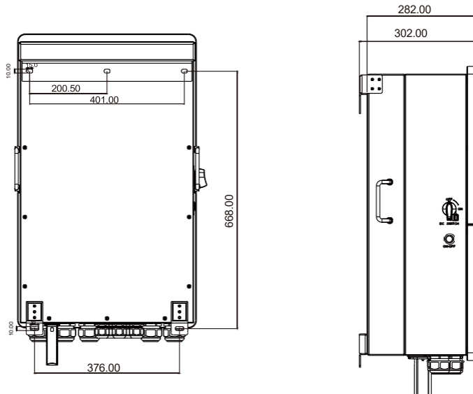
Розміри інвертора
