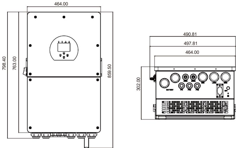
Розміри інвертора
